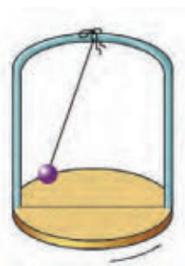
pendulum
