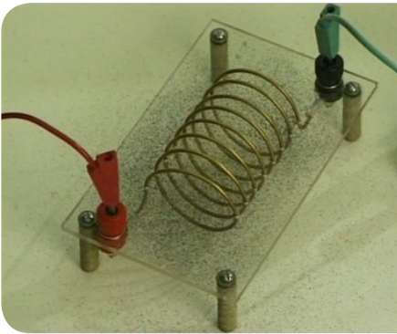
Мал. 17.2. Дослідження магнітного поля котушки зі струмом:
