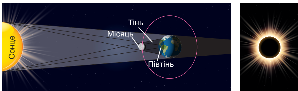
Мал. 24.6. Схема сонячного затемнення (примітка: масштаб відстаней та розмірів на малюнку не дотримано)
