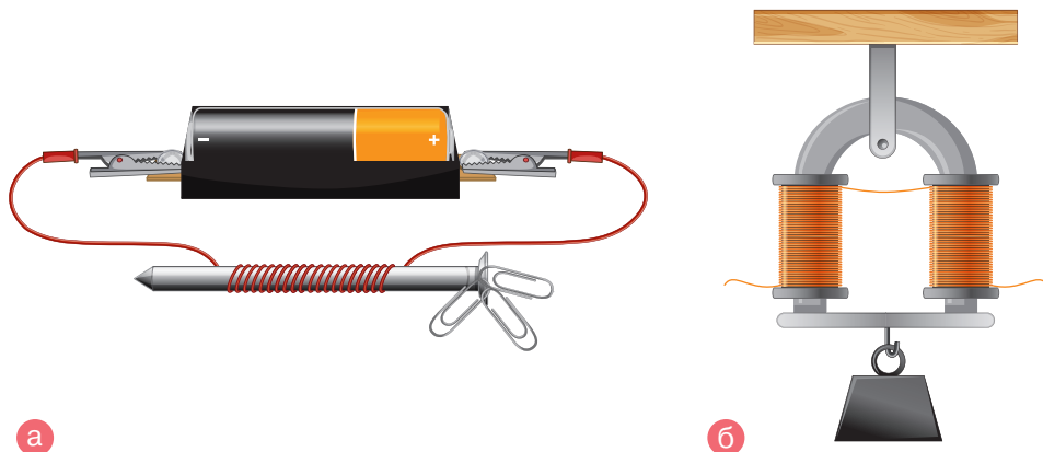
Мал. 17.7. Електромагніти: а — саморобний електромагніт; б — модель електромагніту підсиленої дії
