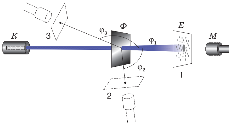
Мал. 30.3. Схема досліду Резерфорда
