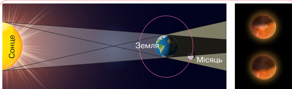
Мал. 24.7. Схема місячного затемнення (примітка: масштаб відстаней та розмірів на малюнку не дотримано)
